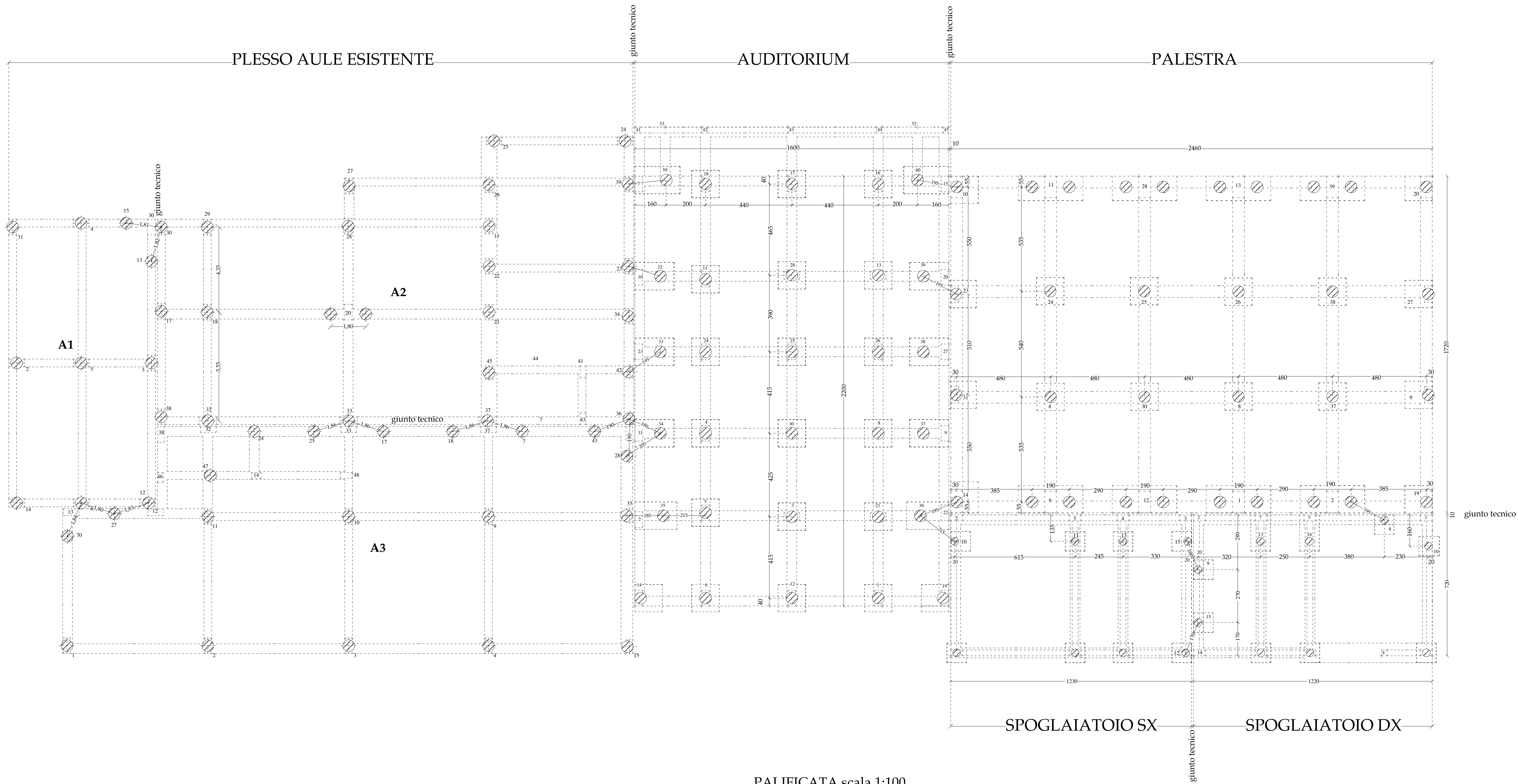
PALIFICATA scala 1:100
